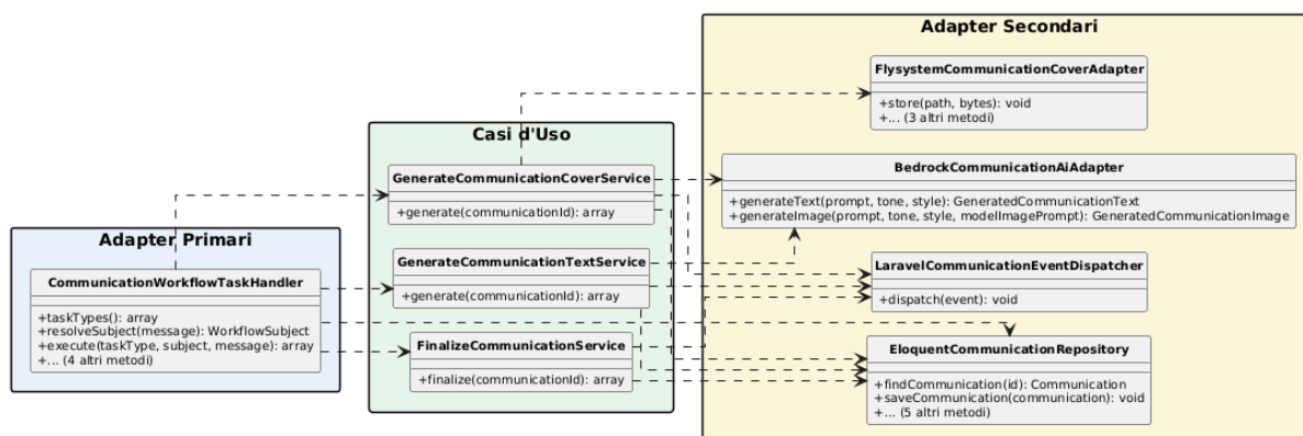
Figura 42: Diagramma classi parziale: Flusso di generazione asincrona
