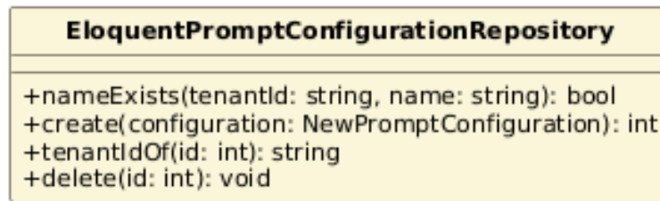
Figura 70: Classe: EloquentPromptConfigurationRepository
